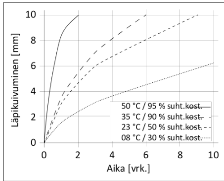
Kaavio 1: Kuivumisnopeus Sikasil® SG-20
