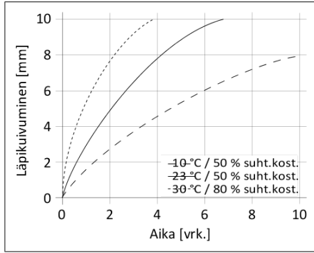
Kaavio 1: Kuivumisnopeus SikaTack® Panel-50
