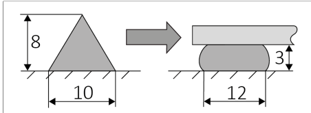
Kuva 1: Ohje liimasauman levitysmuodoksi ja puristamiseksi lopulliseen muotoon.
